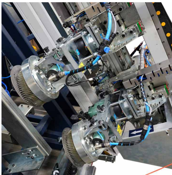
fot. gwoździarki BIZON 903DC JUMBOv3 na moście maszyny Callisto 6
